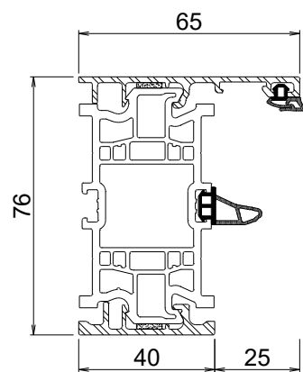
Telaio L
