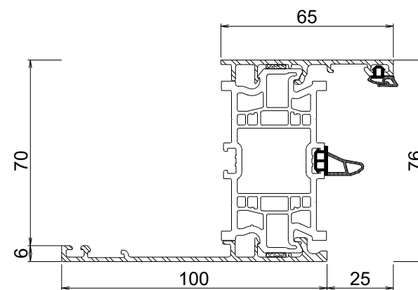
Telaio Z60
