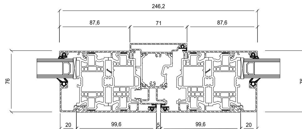
Nodo centrale - anta maggiorata, doppio vetro
