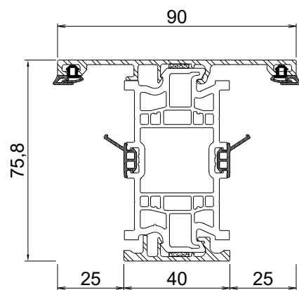
Traverso tagliavetro
