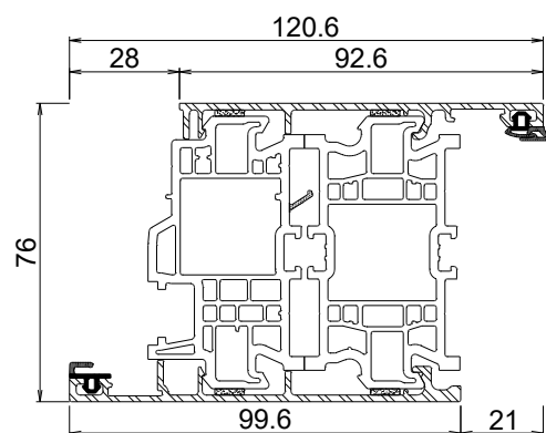
Anta maggiorata
