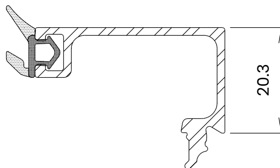
Fermavetro
