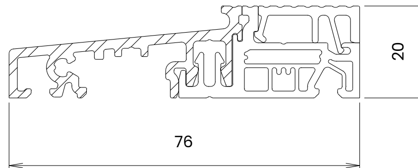
Soglia
