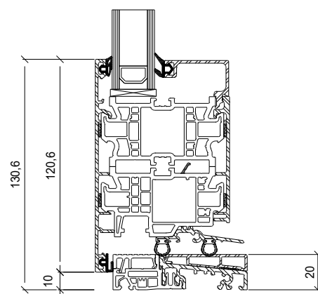
Sezione verticale
