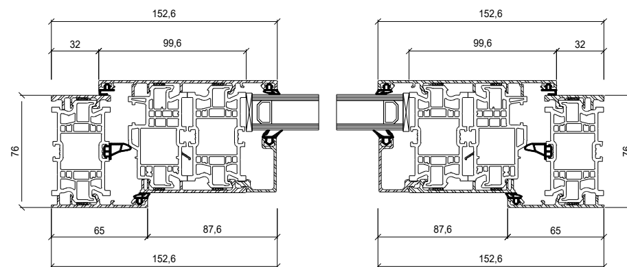
Sezione orizzontale
