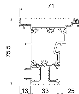
Scambio battuta
