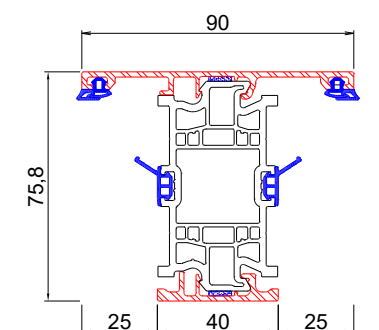
Traverso tagliavetro
