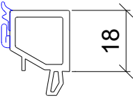
Fermavetro squadrato
