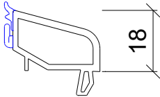
Fermavetro arrotondato
