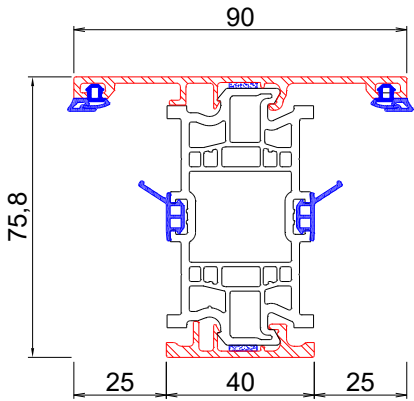
Traverso tagliavetro
