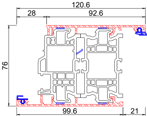
Anta maggiorata
