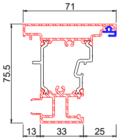
Scambio battuta
