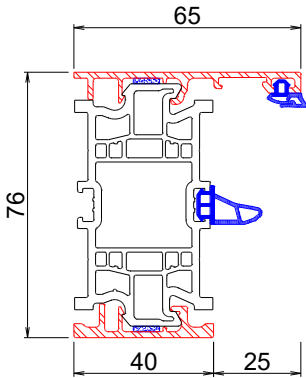
Telaio L
