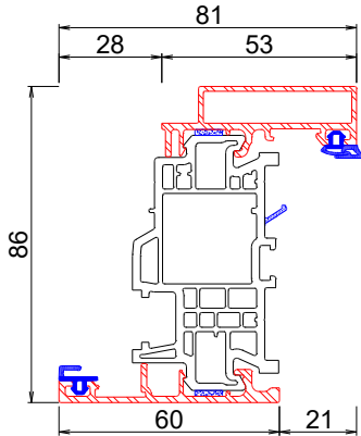
Anta complanare
