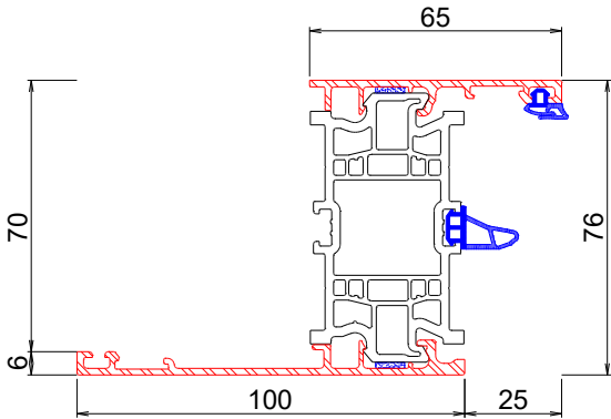
Telaio Z60
