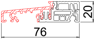
Soglia
