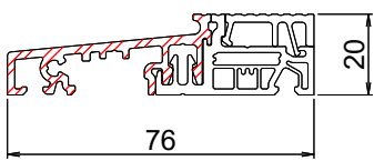
Soglia 20 mm
