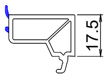
Fermavetro Squadrato
