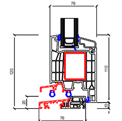
Anta Maggiore
