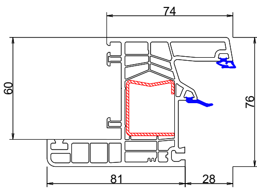
Telaio Z35
