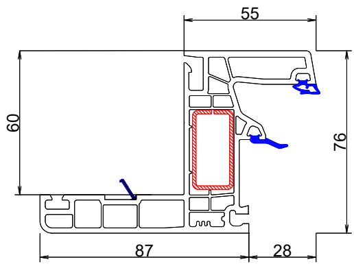
Telaio Z60
