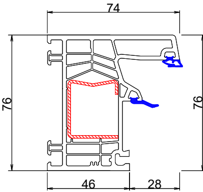
Telaio L
