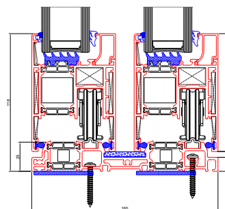
Nodo inferiore
