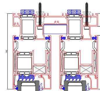
Nodo superiore
