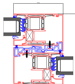
Nodo centrale
